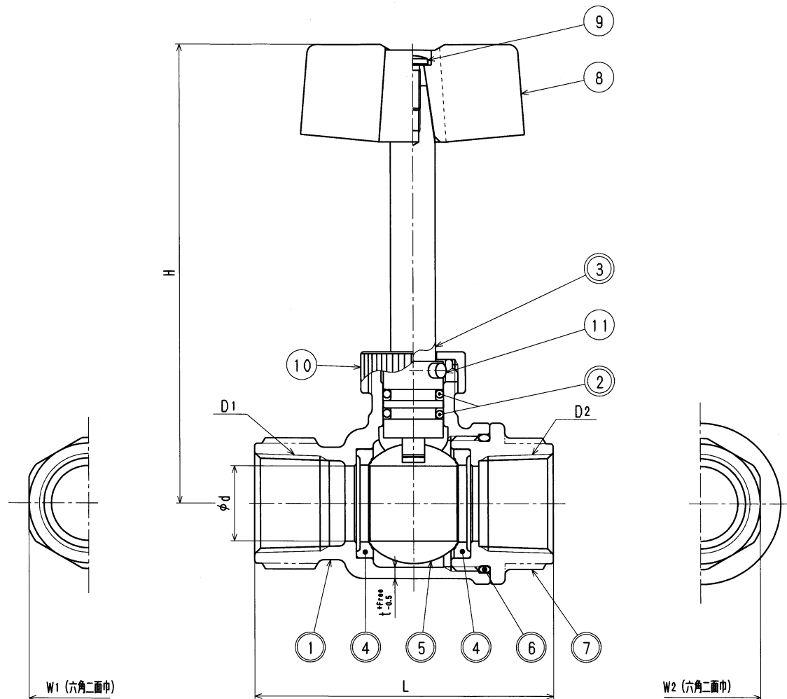
寸法表
